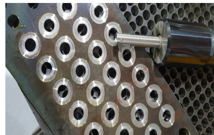
After back spot-faced test (hole \Phi 13.1 _ spot faced \Phi 26.2 ) 백 페이싱 테스트후의 사진 (홀 \Phi 13.1 , 페이싱 \Phi 26.2 )
